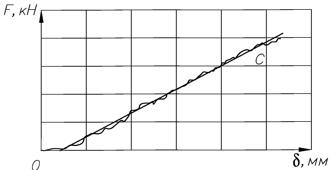
Рисунок А.14 — Кривая нагружения – деформации
