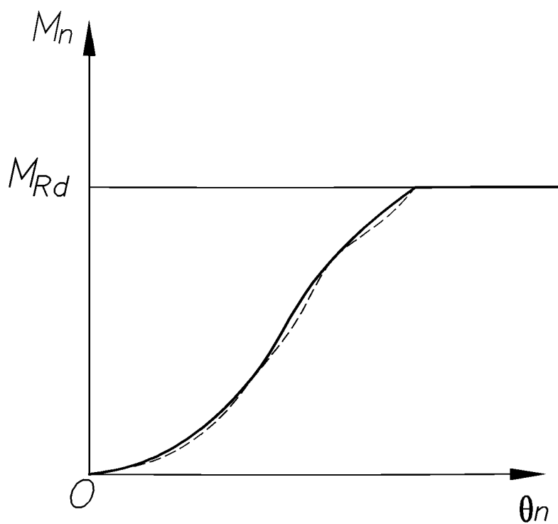
Рисунок А.8 — Типовая линейаризация средней кривой
