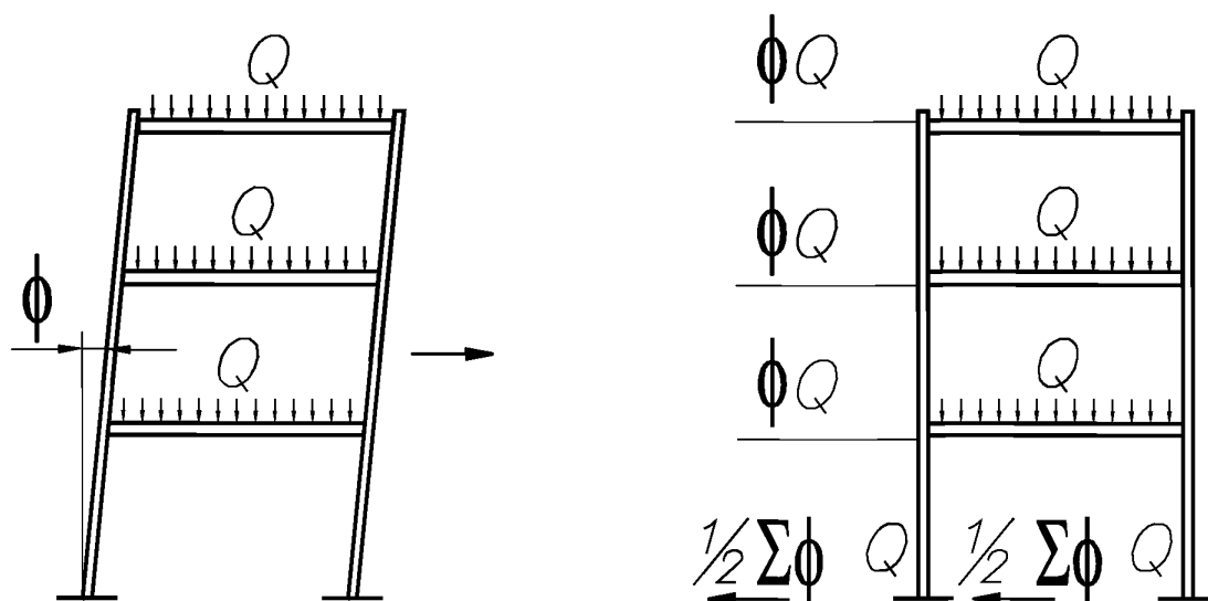
Рисунок 7 — Эквивалентные горизонтальные усилия
