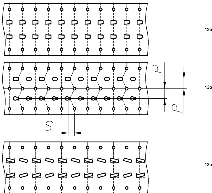
а) нешахматное расположение отверстий; б) шахматное расположение отверстий; с) наклонные отверстия
