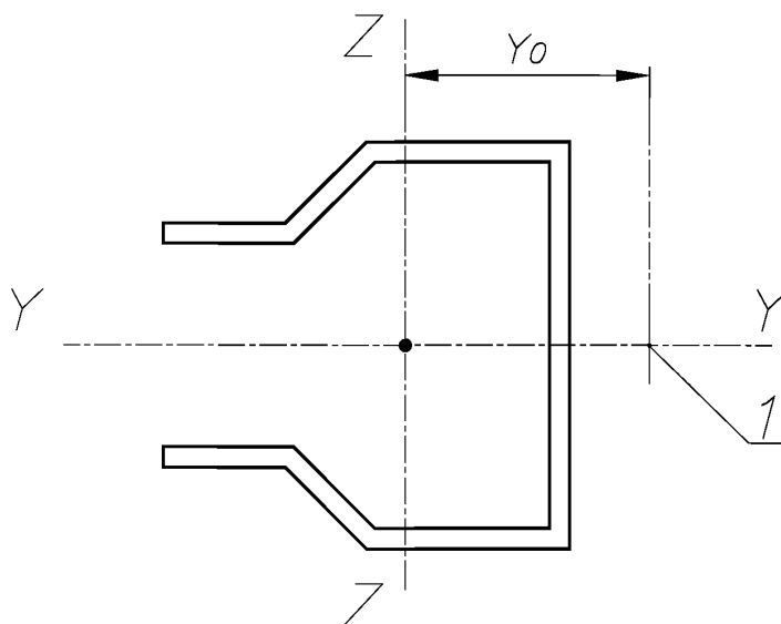
1 — центр изгиба сечения
