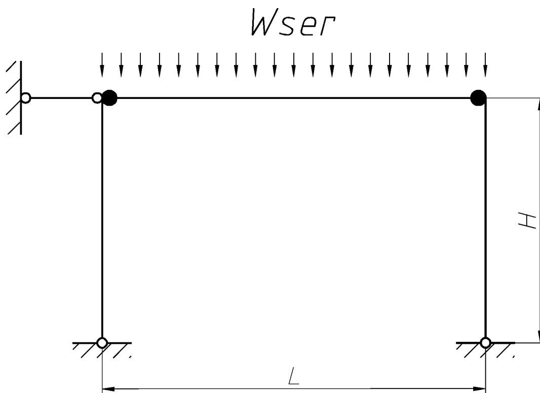
Рисунок 18 — Схема для предварительного расчета прогиба балки
