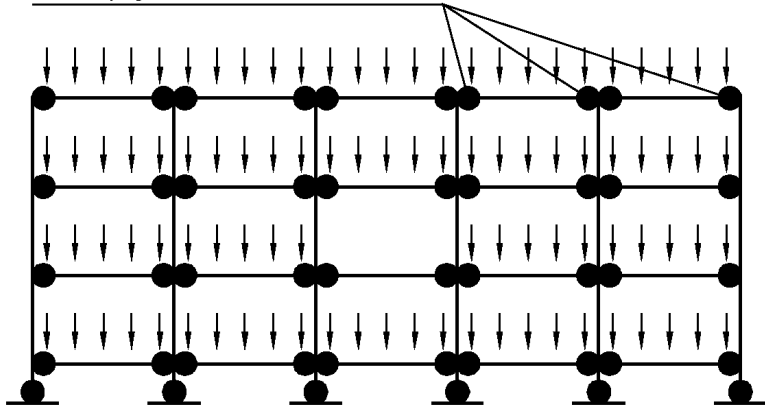
Рисунок 27 — Схемы нагружения для расчета в X-направлении
